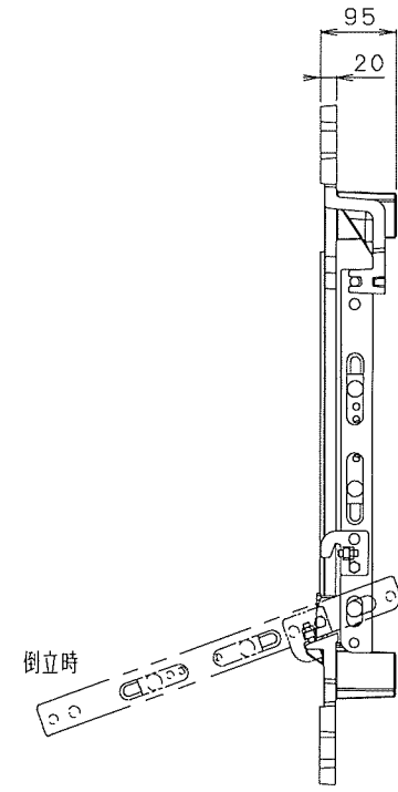
A-A断面図
